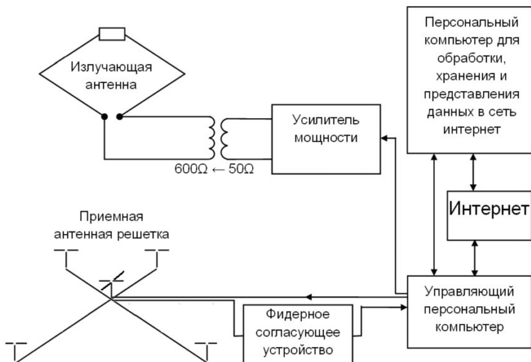
Рис. 1. Структурная схема сетевого ионозонда «ТОМИОН»
