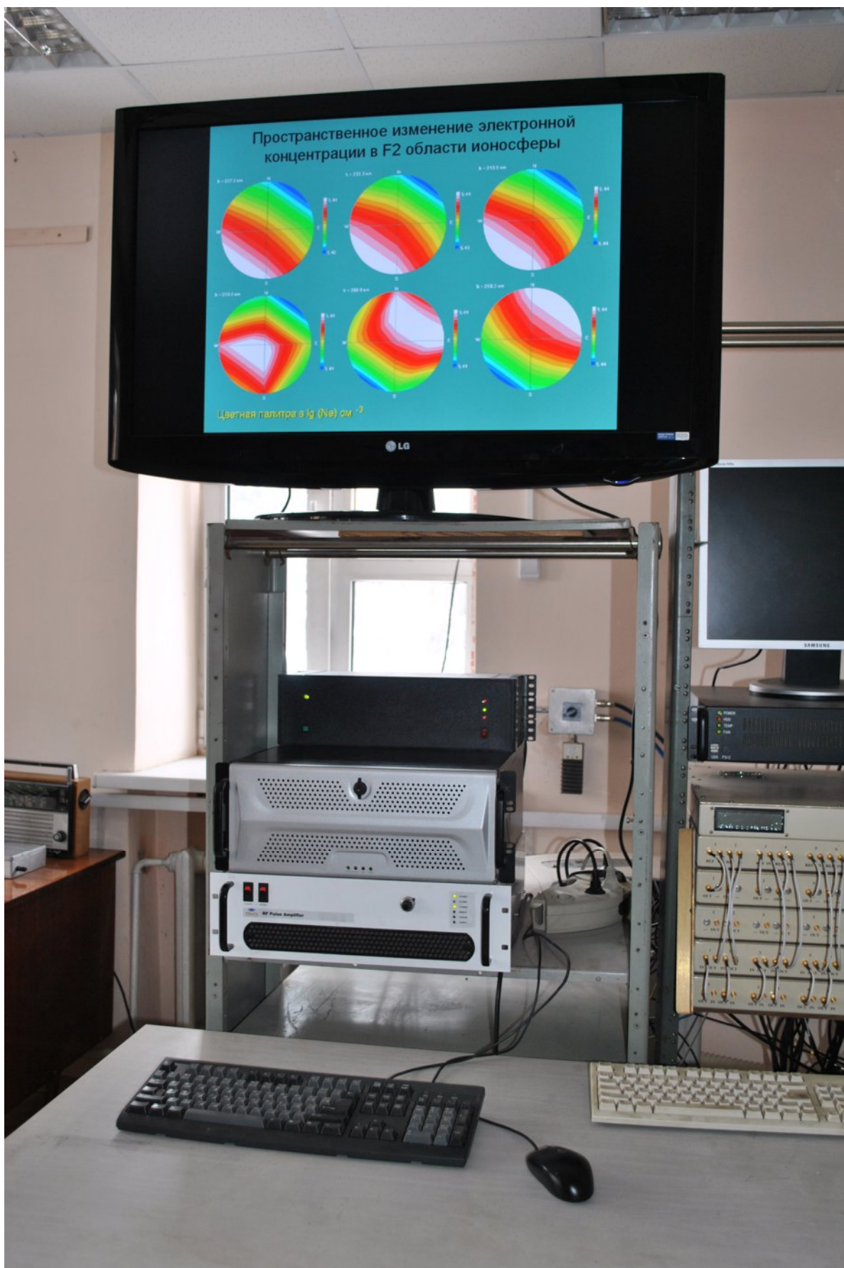
Рис. 2. Лицевая сторона ионозонда «ТОМИОН»
