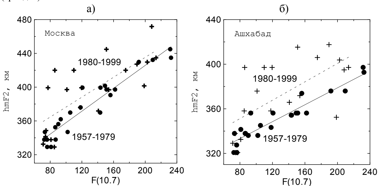
Рис. 6. Изменение со временем величины hmF2 для станций Москва (а) и Ашхабад (б) согласно работе [Данилов и Ванина-Дарт, 2010б]. Точки и сплошная прямая относятся к 1957-1979 гг., а кресты и штриховая прямая – к 1980-1999 гг.
