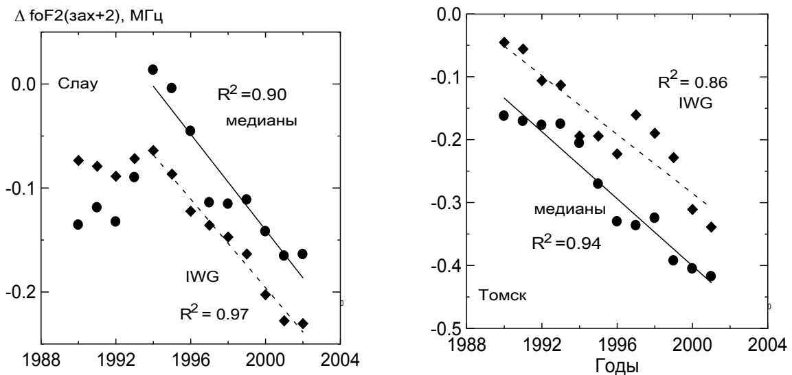
Рис.11. Изменение со временем величины foF2(\text{зах}+2) для станций Слау и Томск по медианным данным и по данным в iwг формате согласно работе [Данилов, 2011б].
