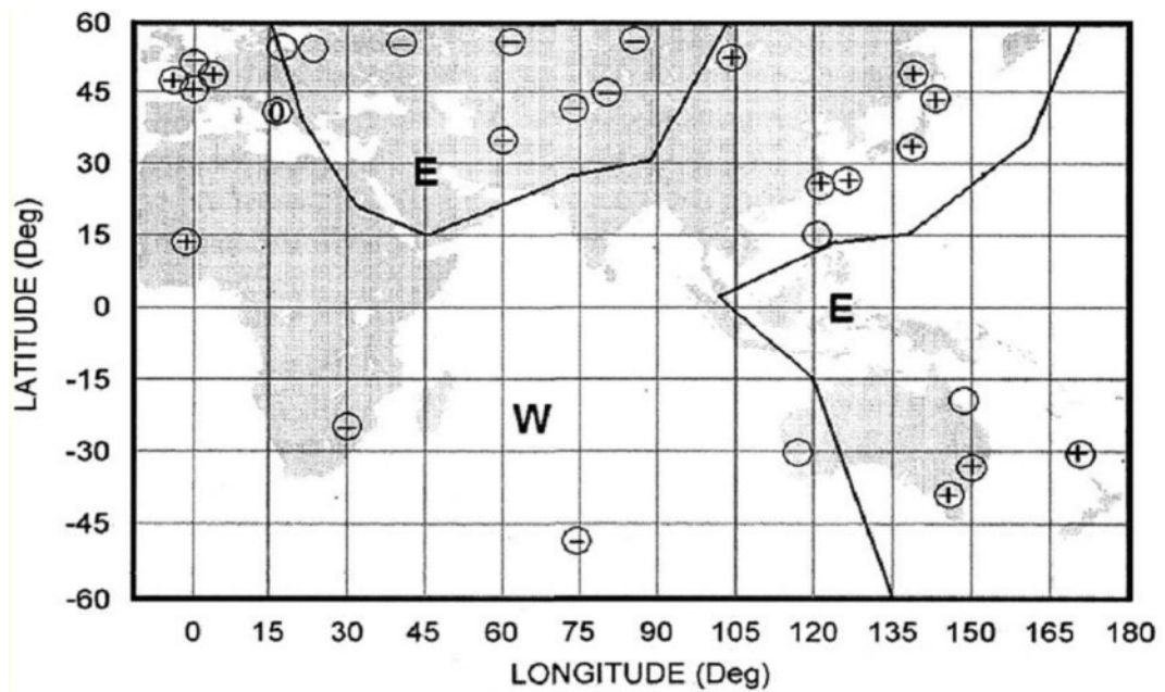
Рис. 5. Карта размещения станций с положительными и отрицательными трендами величины foF2(02)/foF2(14) из работы [Danilov, 2008a].
