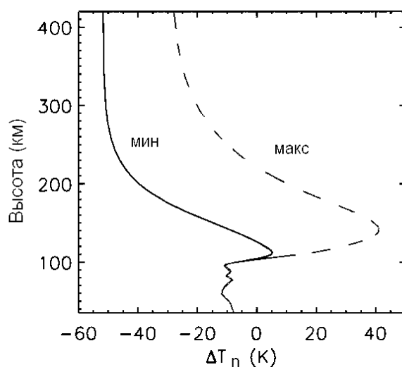
Рис. 15. Высотный профиль ожидаемого уменьшения нейтральной температуры T_n согласно модельным расчетам [Qian et al., 2011].
