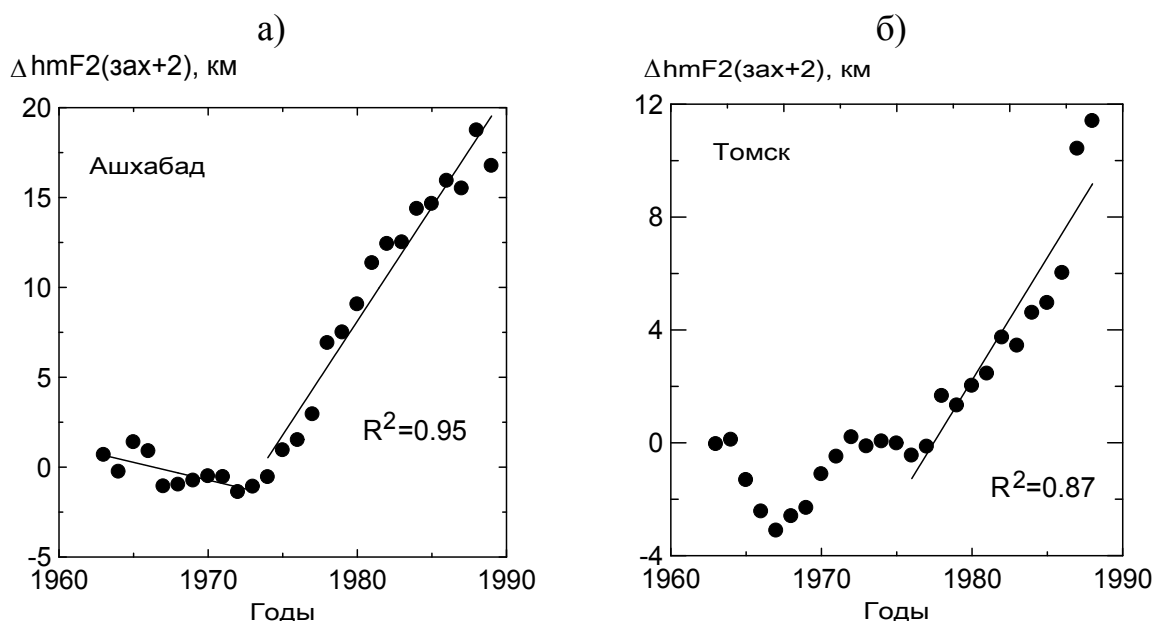
Рис. 8 Зависимость величины hmF2(зах+2) от солнечной активности для Ашхабада (а, июнь-июль) и Томска (б, январь-февраль) согласно работе [Данилов и Ванина 2010б].
