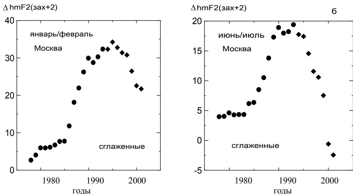
Рис. 9. Изменение со временем высота слоя F2 согласно данным станции Москва.
