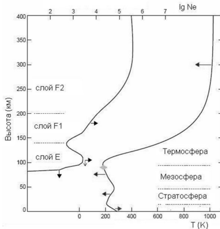
Рис. 1 Схема изменений в температуре и электронной концентрации согласно [Lastovicka et al., 2008].
