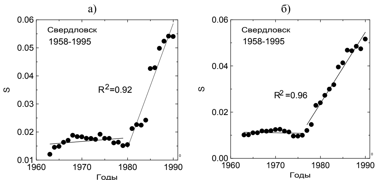
Рис. 7. Зависимость величины S от времени для станции Свердловск в январе-феврале (а) и июне-июле (б) согласно работе [Данилов и Ванина-Дарт, 2010а].
