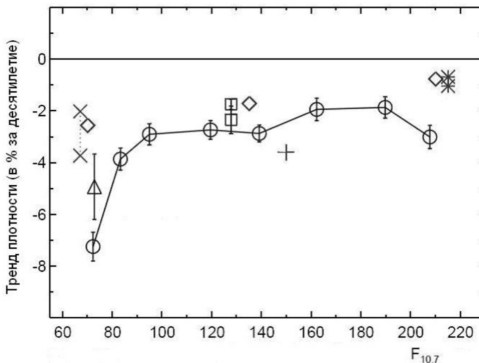
Рис. 3 Изменение плотности термосферы при различных уровнях солнечной активности согласно экспериментальным данным (треугольники - Keating et al. [2000], 360 км; кружки - Emmert et al. [2004], 530 км; квадраты - Markos et al., [2005], 390 км) и теоретическим моделям (косые кресты – Roble and Dickinson [1989], 400 км; звездочки – Rishbeth and Roble [1992], 400 км; прямые кресты – Akmaev et al. [2006], 200 км; ромбы – Qian et al. [2009], 400 км) из работы [Lastovicka, 2009].
