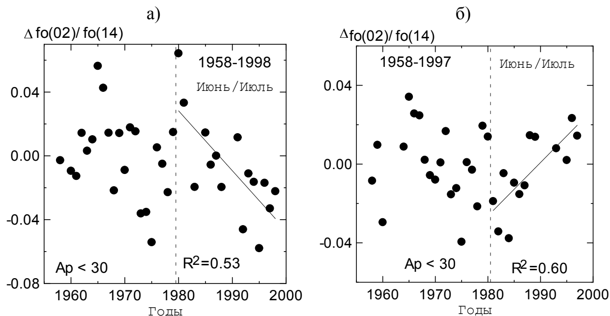
Рис. 4 Изменение отношения foF2(02)/foF2(14) со временем для станций Ленинград (а) и Пуатье (б) согласно работе [Данилов и Ванина-Дарт, 2010б].
