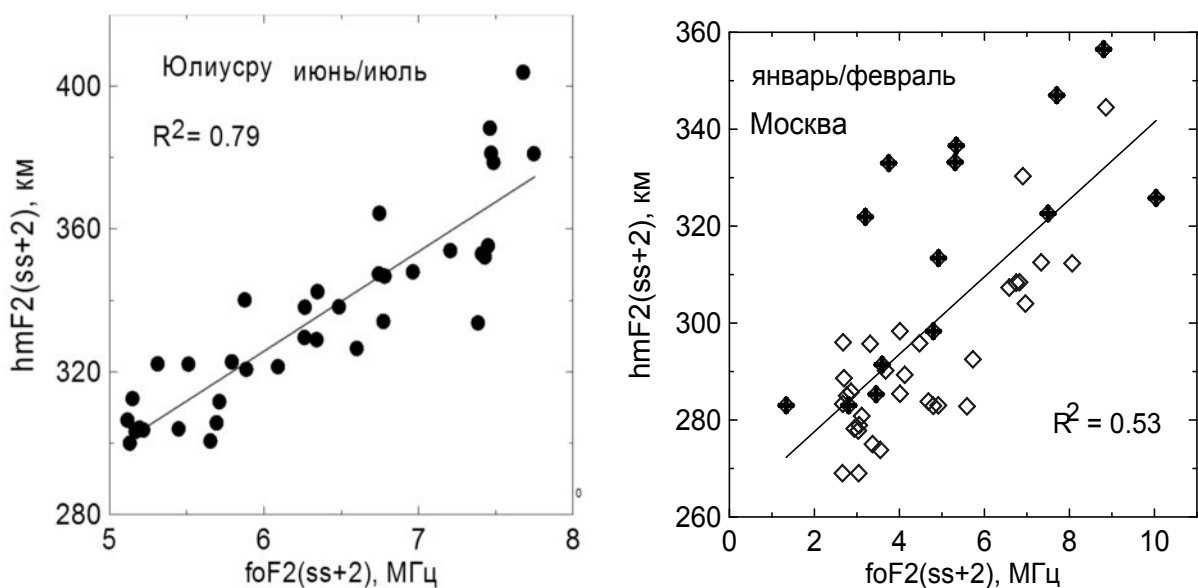
Рис. 10. Связь между hmF2(зах + 2) и foF2(зах + 2) для станций Юлиусру (июнь-июль) и Москва (январь-февраль) согласно работе [Данилов и Ванина 2010в].
