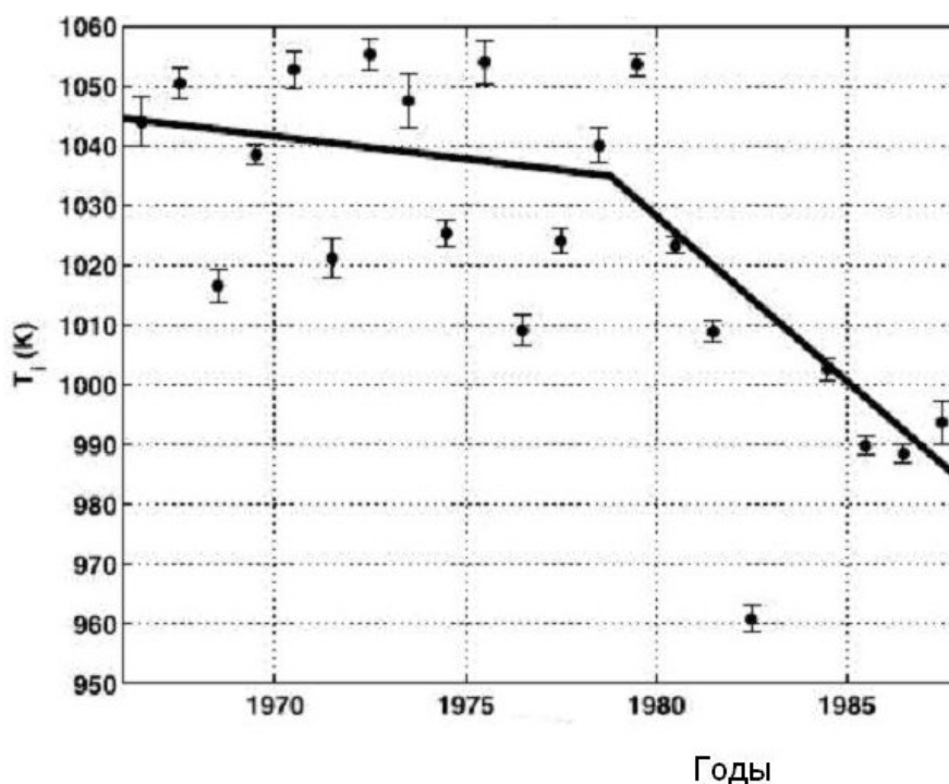
Рис. 12. Изменение температуры ионов по измерениям методом НР согласно [Donaldson et al., 2010].
