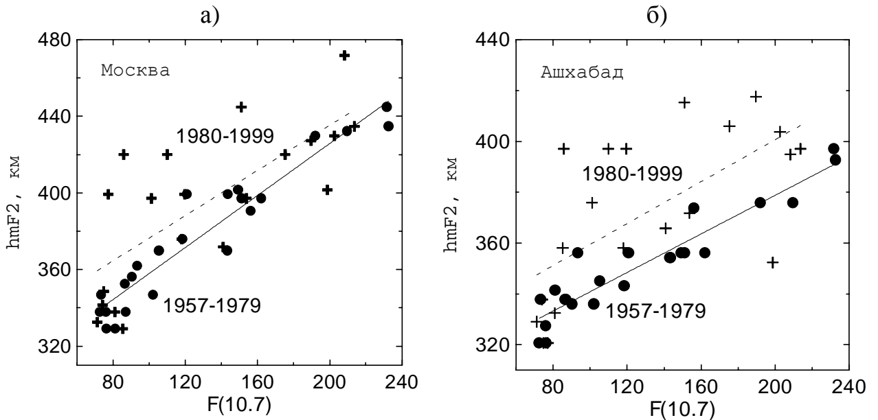
Рис. 6. Изменение со временем величины hmF2 для станций Москва (а) и Ашхабад (б) согласно работе [Данилов и Ванина-Дарт, 2010б]. Точки и сплошная прямая относятся к 1957-1979 гг., а кресты и штриховая прямая – к 1980-1999 гг.
