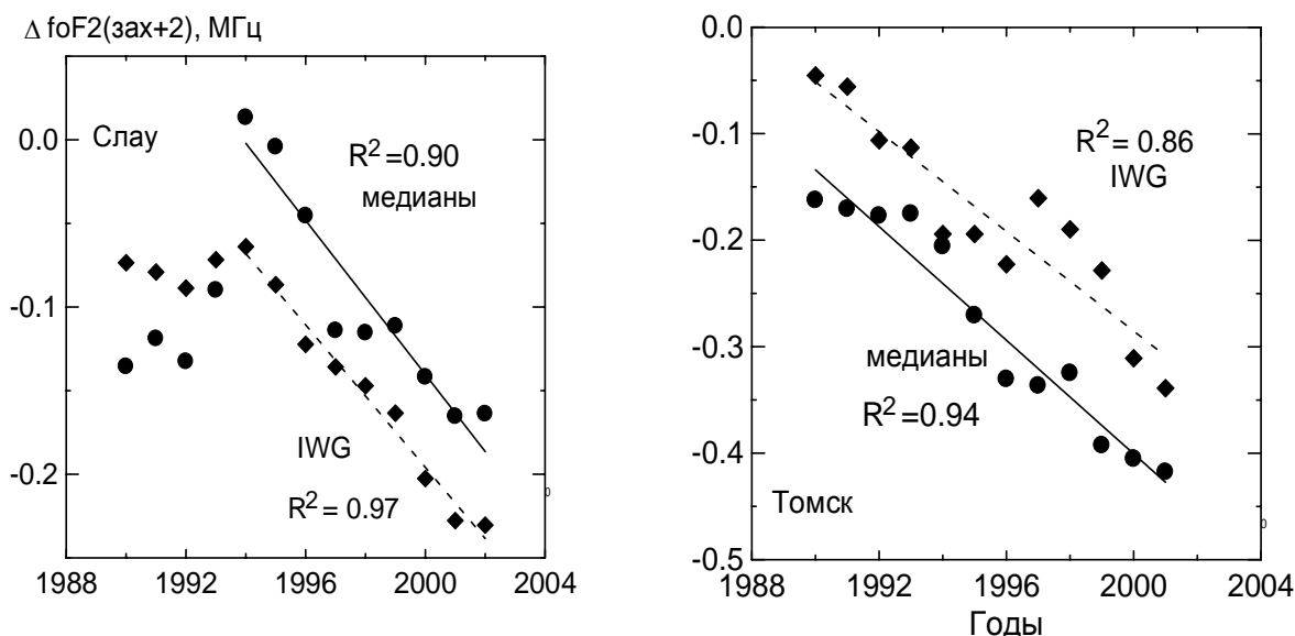
Рис.11. Изменение со временем величины foF2(\text{зах}+2) для станций Слау и Томск по медианным данным и по данным в iwg формате согласно работе [Данилов, 2011б].
